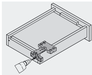
Boren van de haakposities
