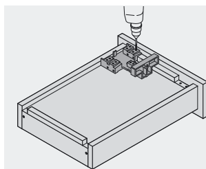
Vorboren van de bevestigingsposities voor de TANDEM-koppeling
